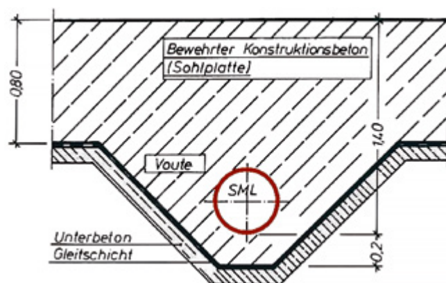
Schnittbild: Voute in einer Betonplatte
